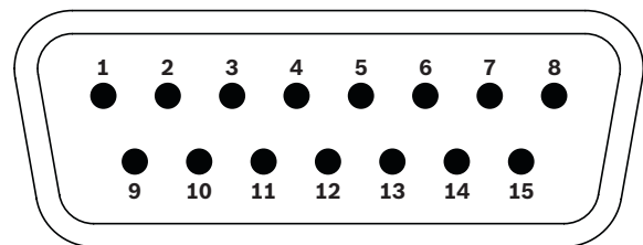
D-Sub 15-polig, Stifte
